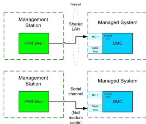
Abbildung 3-2. IPMI Shell-Diagramm
