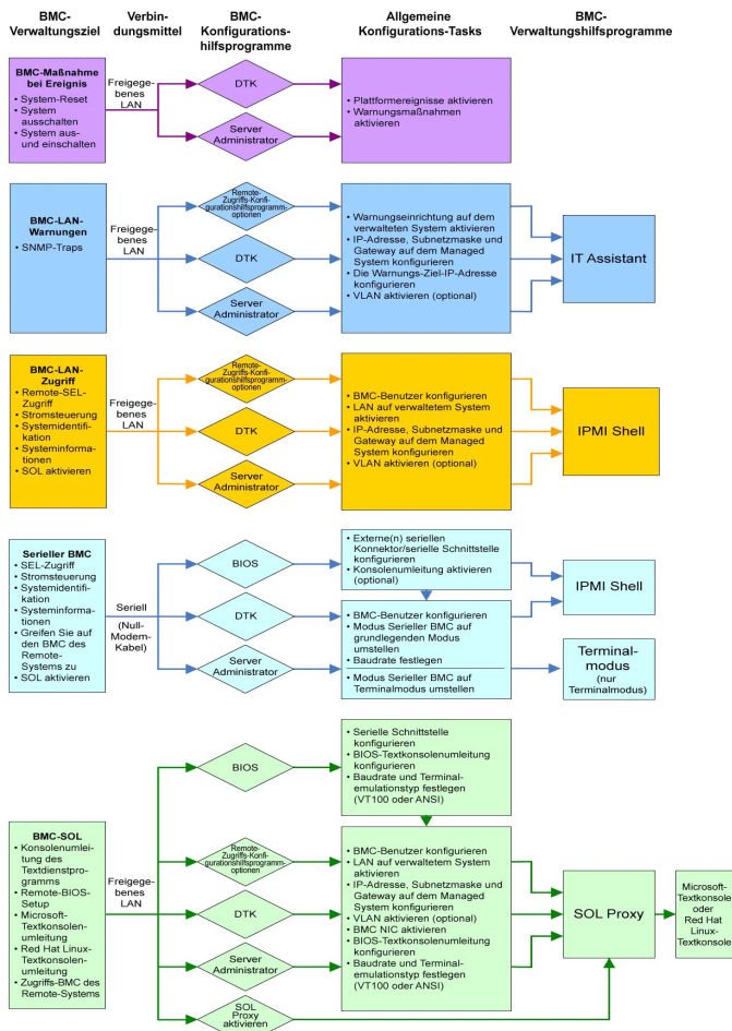
Abbildung 1-1. BMC-Konfigurationsmatrix
